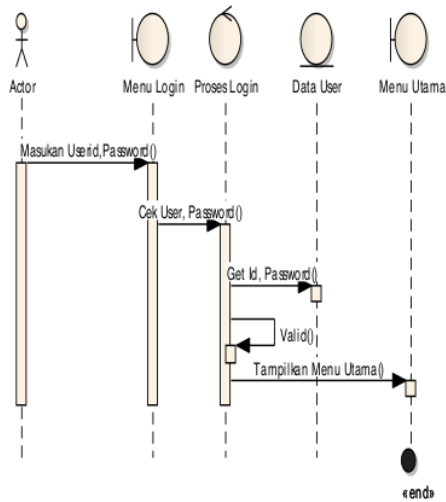
Gambar 3 Sequence Diagram Melakukan Login
