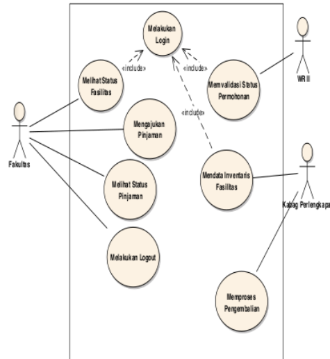
Gambar 2 Use Case Diagram Sistem Baru
