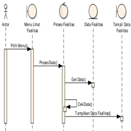
Gambar 4 Sequence Diagram Melihat Status Fasilitas
