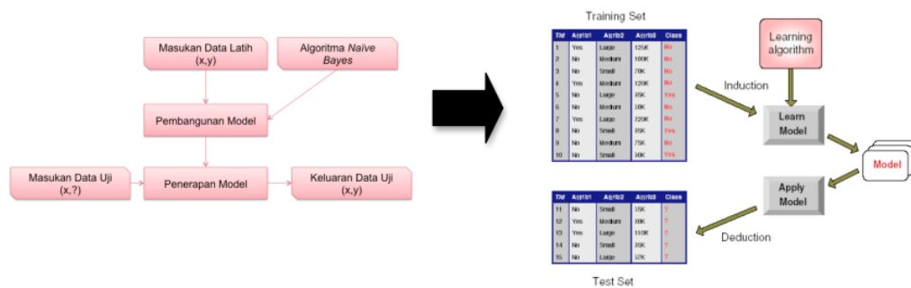
Gambar 4. Proses Pengerjaan Klasifikasi Naïve Bayes
